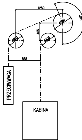
SCHEMAT OLINOWANIA
